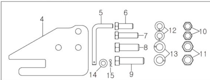
FIG 001 SUB FRAME
